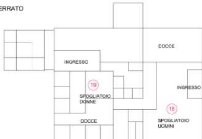
PIANTA PIANO TERRA RIALZATO
